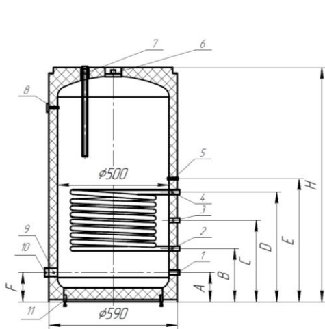
Рис. 1 Бак 150-200-300 литров
