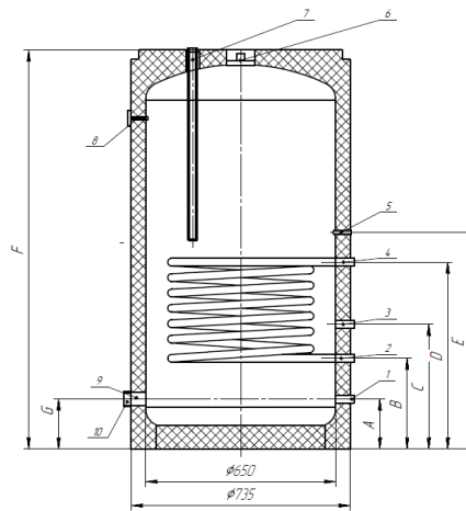
Рис. 2 Бак 400-500 литров
