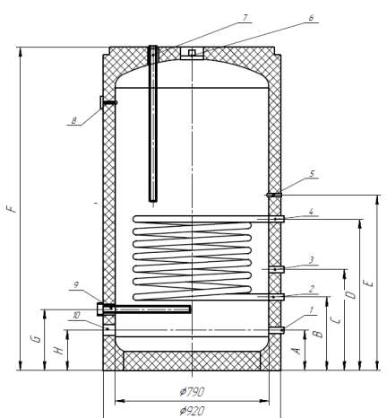
Рис. 3 Бак 750-1000 литров
